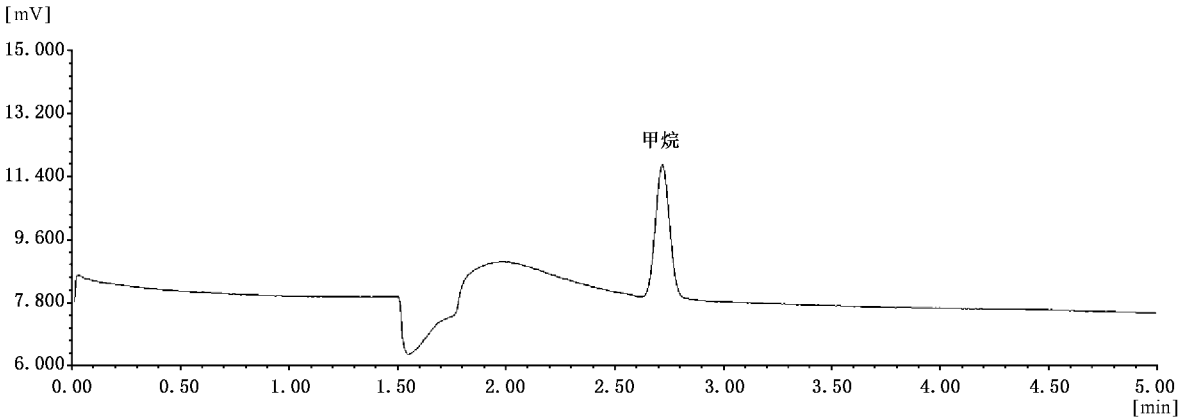
图 A.2 典型标准样品色谱图
