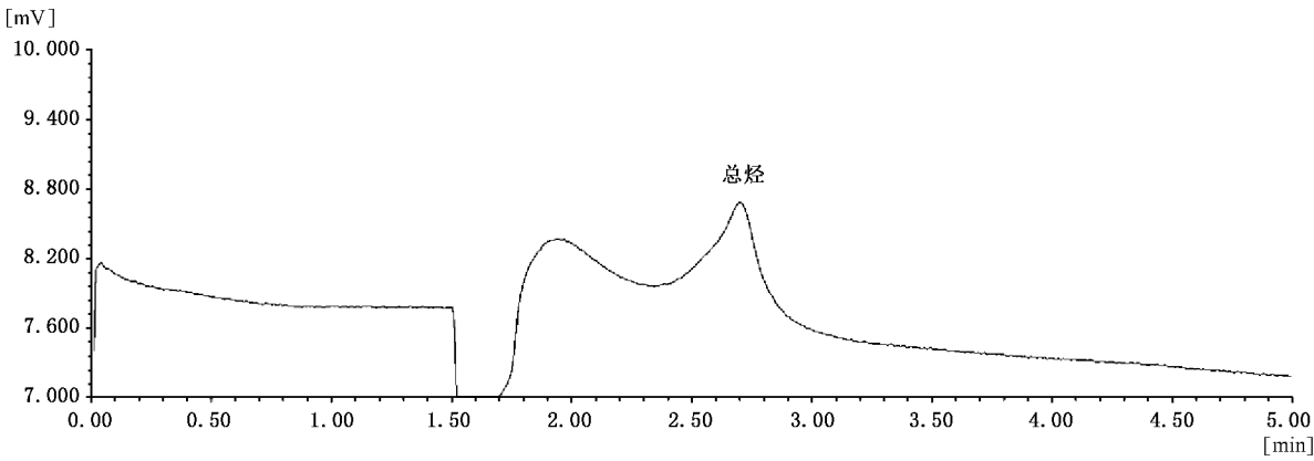
图 A.3 典型样品色谱图
