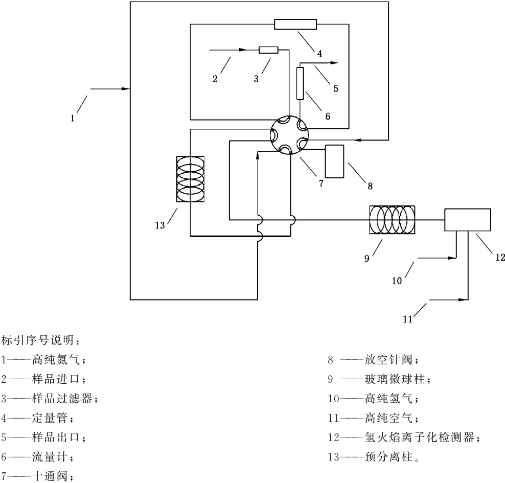
图 A.1 测定总烃的气路流程示意图
